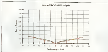
Gerade Kennlinie, identische Kräfte auf jeder Achse, Position kraftmäßig schlecht zu unterscheiden.
